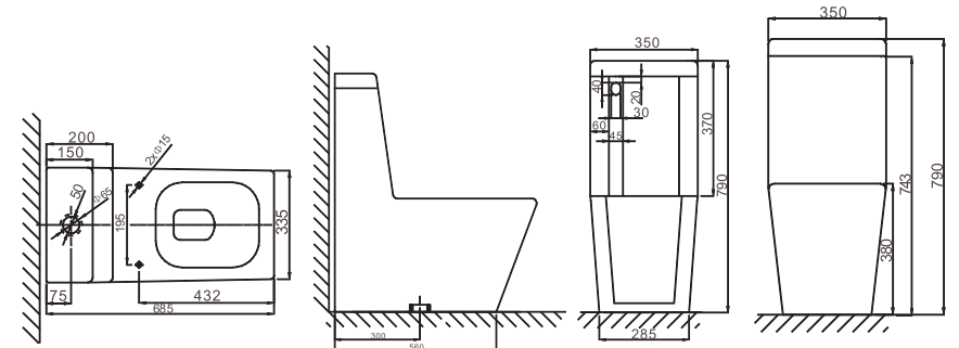
CO-1012 Unit:mm
