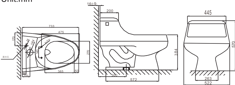
CO-1013 Unit:mm
