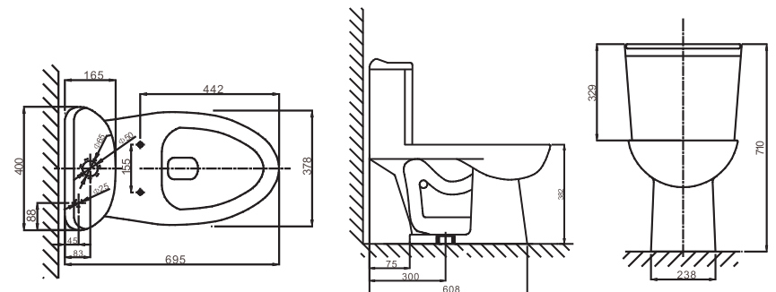
CO-1010 Unit:mm
