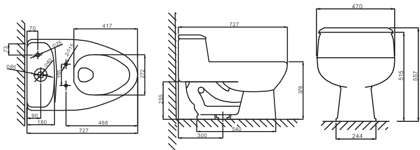
CO-1017 Unit:mm
